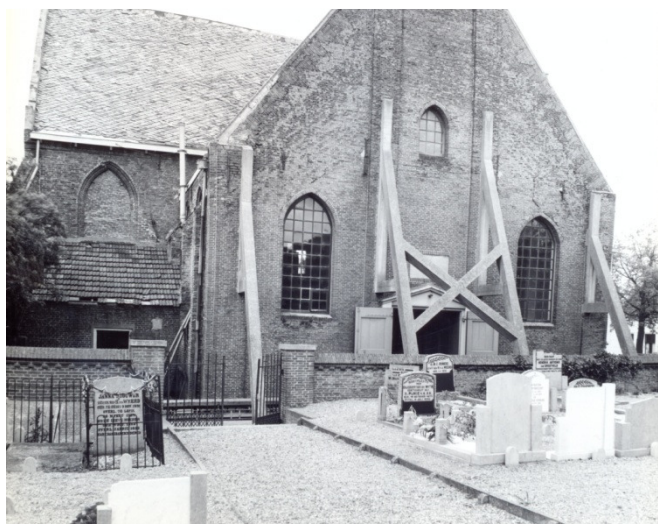
Afbeelding 3. De betonnen steunberen om de toren te ondersteunen.
