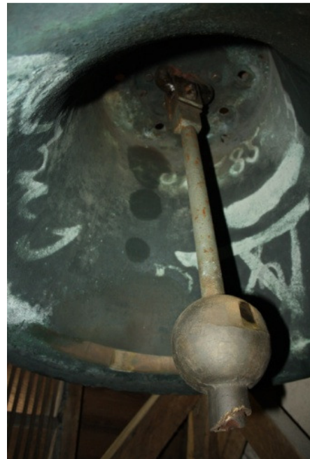
Afbeelding 2. De klepel, met afgebroken klepelstaart.
